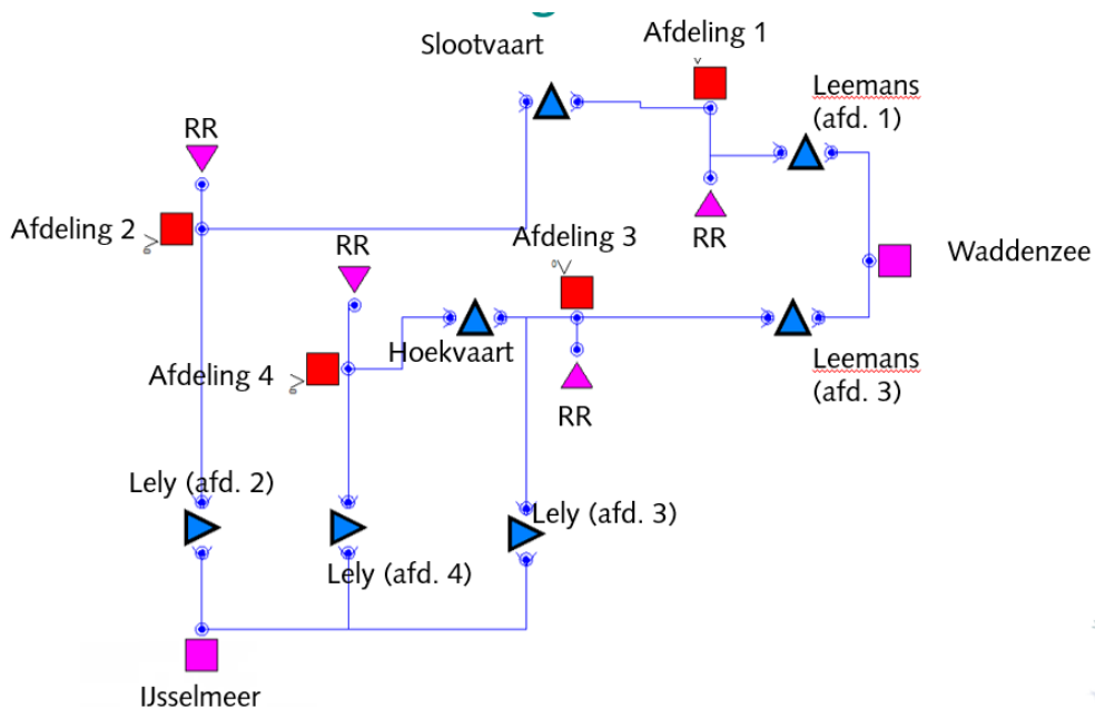
SCHEMATISATIE VAN DE WIERINGERMEERPOLDER IN RTC-TOOLS
