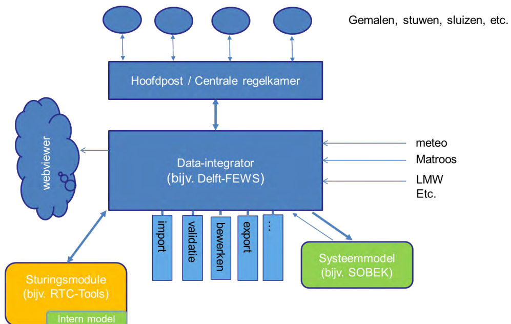
FIGUUR 2.1 ELEMENTEN IN EEN OPERATIONEEL WATERBEHEERSYSTEEM
